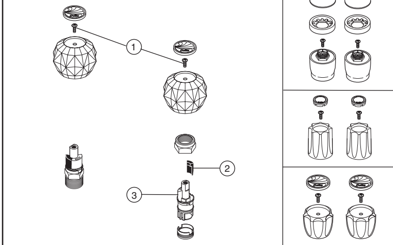
Knob Handles/Manijas de Perilla/Poignées Sphériques
